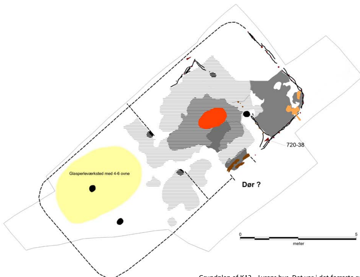
Grundplan af K12 – Lyrens hus. Det var i det forreste rum at de fleste ting var efterladt. I midten ses ildstedet og bagerst i huset har perlemageren arbejdet. Tegning: Museum Vest.
