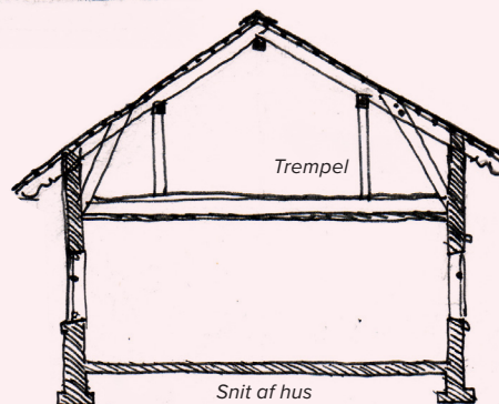
Snit af hus
